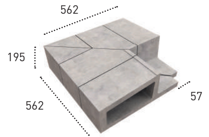
ESQUINA INTERIOR Ref. SISTEMA BLOCK EI 25
