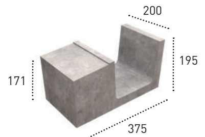
3 PIEZA BLOCK 25 MACIZA CORTADA Ref. SISTEMA BLOCK 25 MEDIO MACIZO
